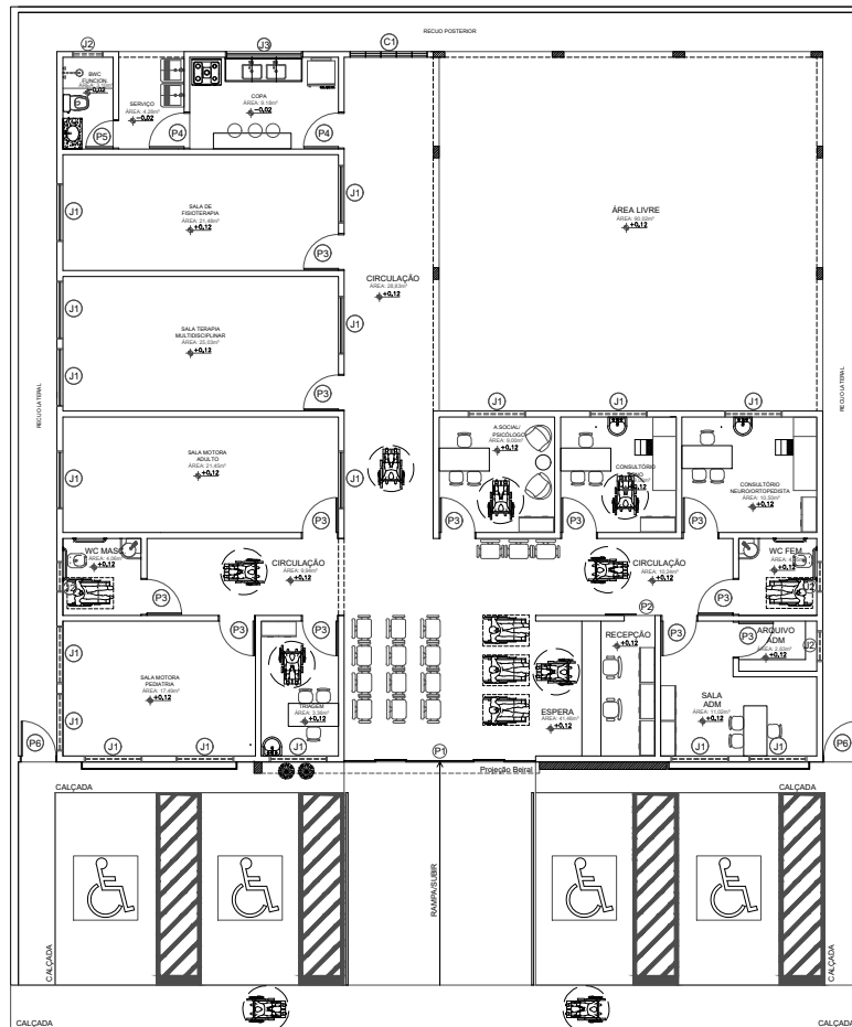
PLANTA DE LAYOUT - CENTRO DE REABILITAÇÃO esc: 1:100
